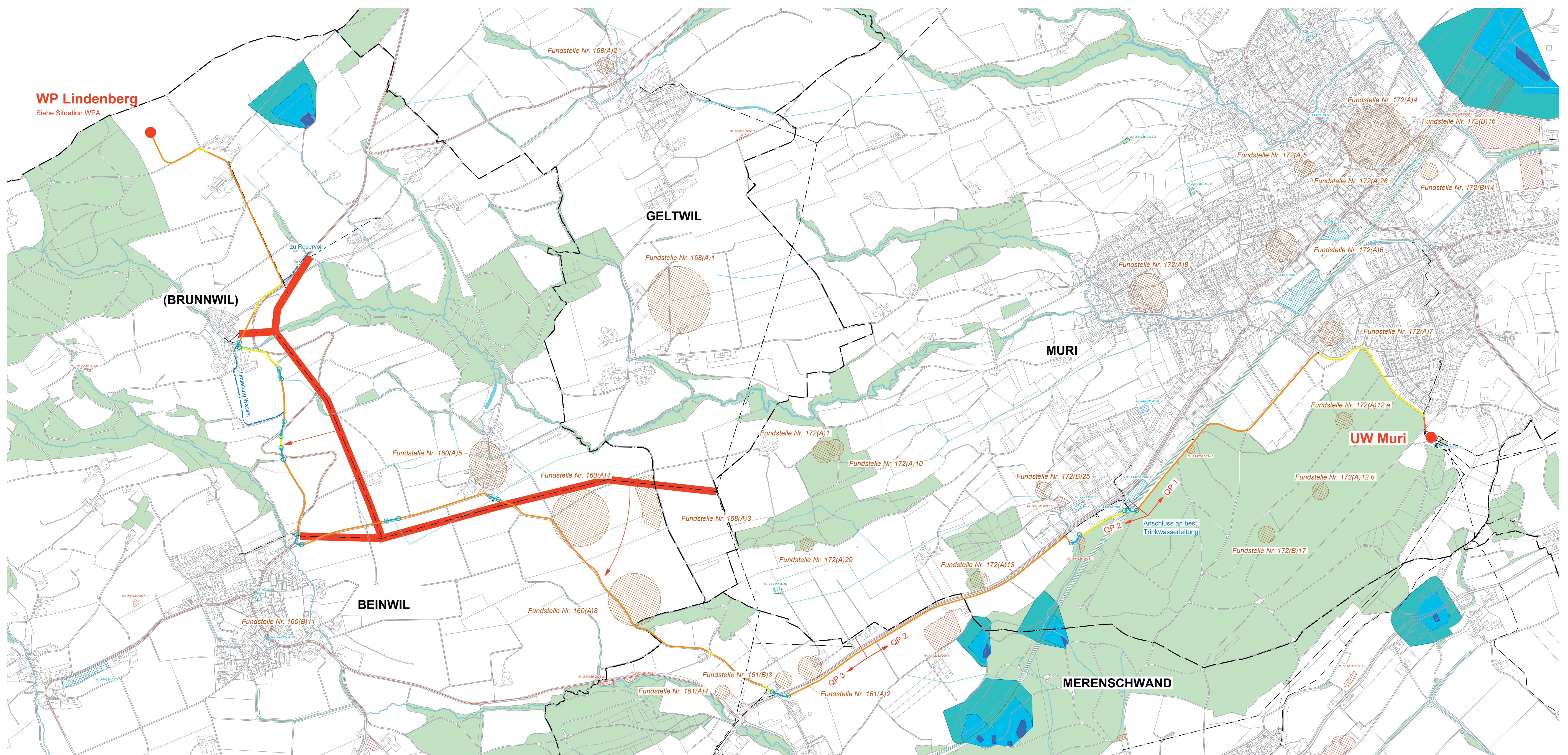
Abb. 1: Lokalisierung der heute bestehenden Mittelspannungsfreileitungen, die erdverlegt werden können. Die Leitungen haben eine Gesamtlänge von rund 3,3 km. Die orange dargestellte Leitungstrasse entspricht der gewählten Variante der Netzanbindung des Windparks. Sie wird ebenfalls erdverlegt. Quelle: AEW Energie AG.
