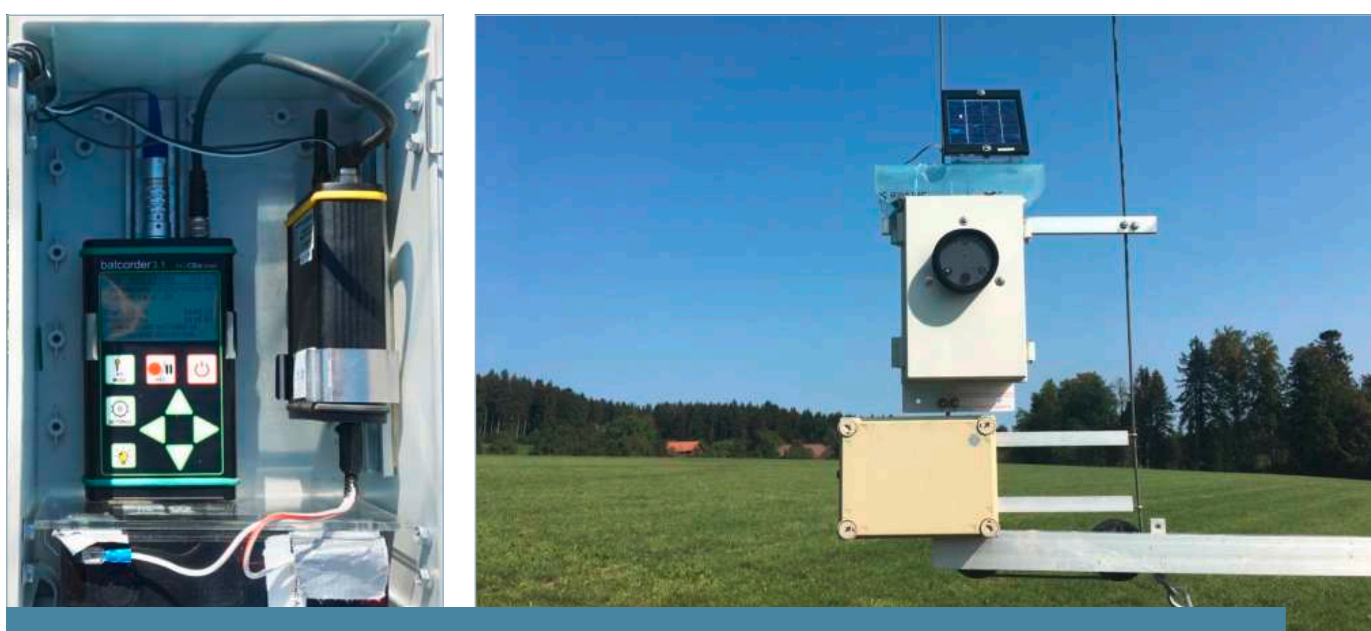
Abb. 1a) Position des Messgerätes auf 88 m. 1b) BatUnit mit Batlogger. 1c) BatUnit von aussen. Das Mikrofon ist die schwarze Scheibe. Quelle: SWILD.
