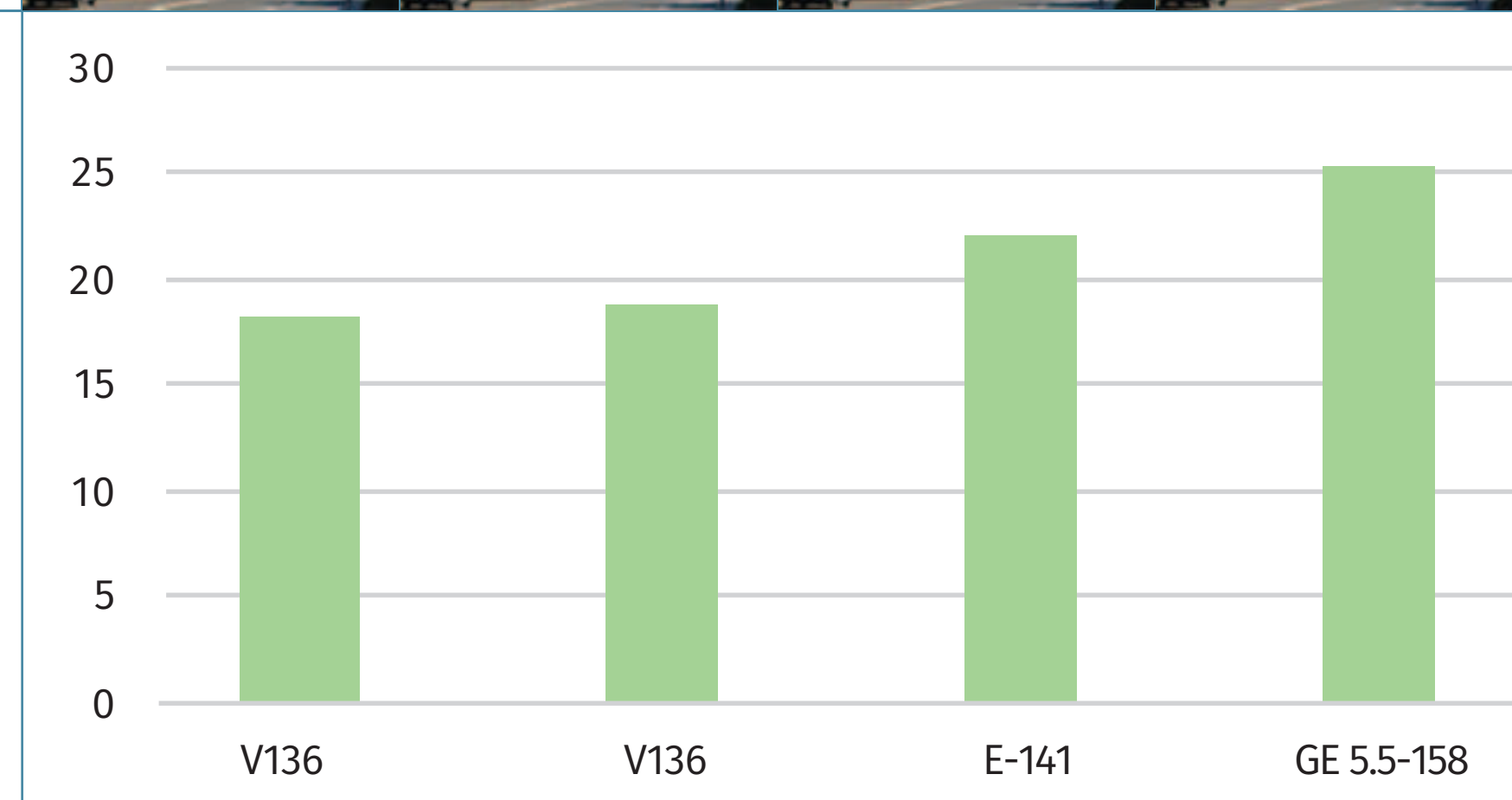
Abb. 4: Darstellung des Energieertrages netto (P75) für verschiedene Anlagentypen mit gleichzeitiger Darstellung der Sichtbarkeit von Beinwil aus. Quelle: Meteotest AG, Windpark Lindenberg AG.
